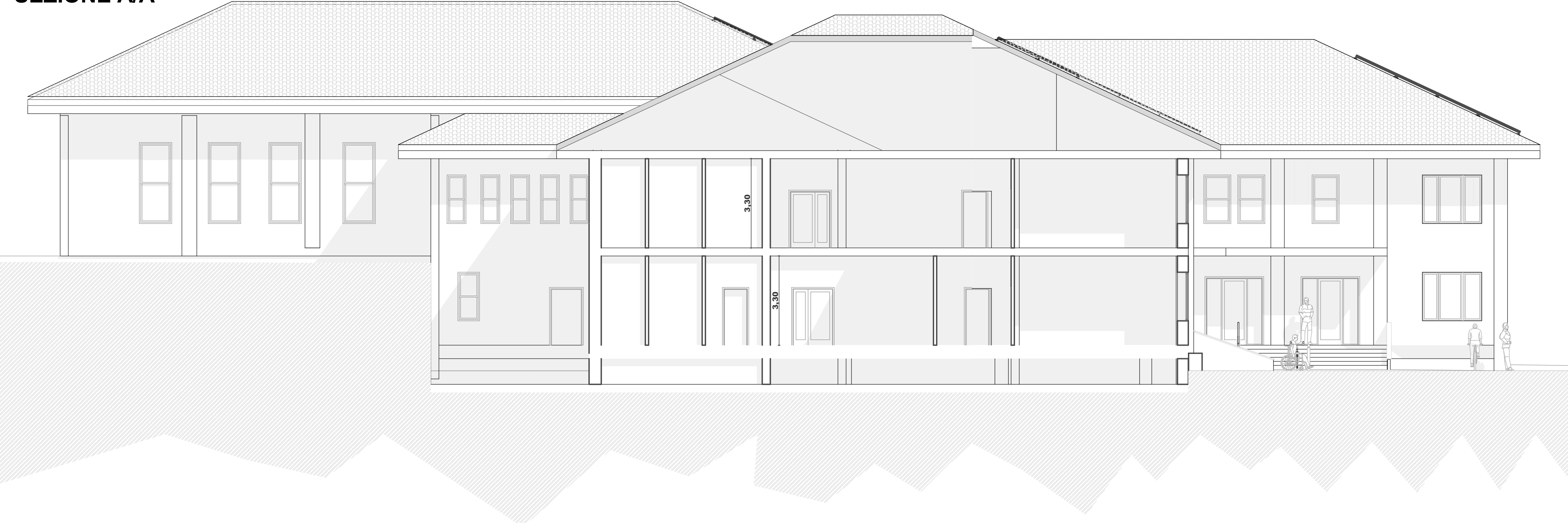
SEZIONE A/A
